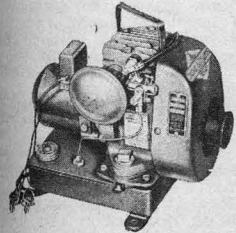
Modelo 100—6 voltios—100 vatios. Amplia capacidad para cargar acumuladores. Pequeño y liviano pero fuerte para el trabajo.
