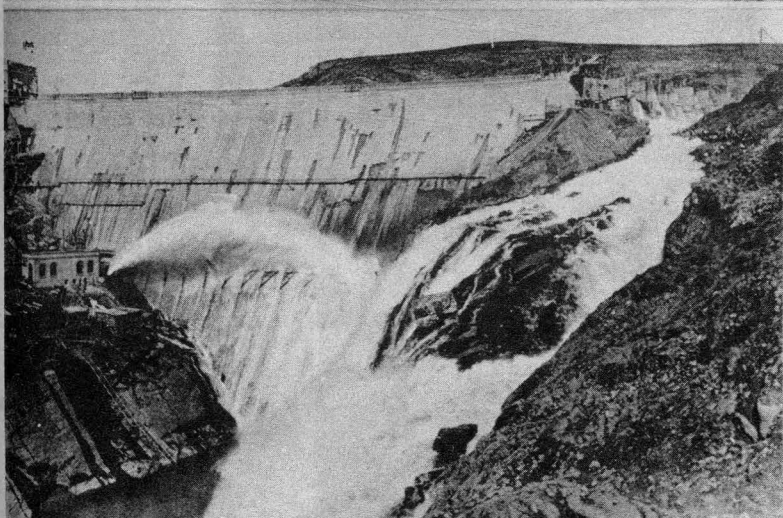
La planta eléctrica y el formidable dique de Lérida, que han sido objeto de bombardeos infructuosos por parte de los aviones del general Franco. Las fábricas de electricidad de Lérida envían diariamente a Barcelona un millón de kilovatios. (Foto International).
