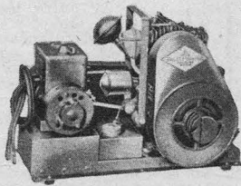
Modelo 200—6 voltios—200 vatios. Arranque eléctrico. Muchas características exclusivas. Doble de capacidad del modelo 100.
